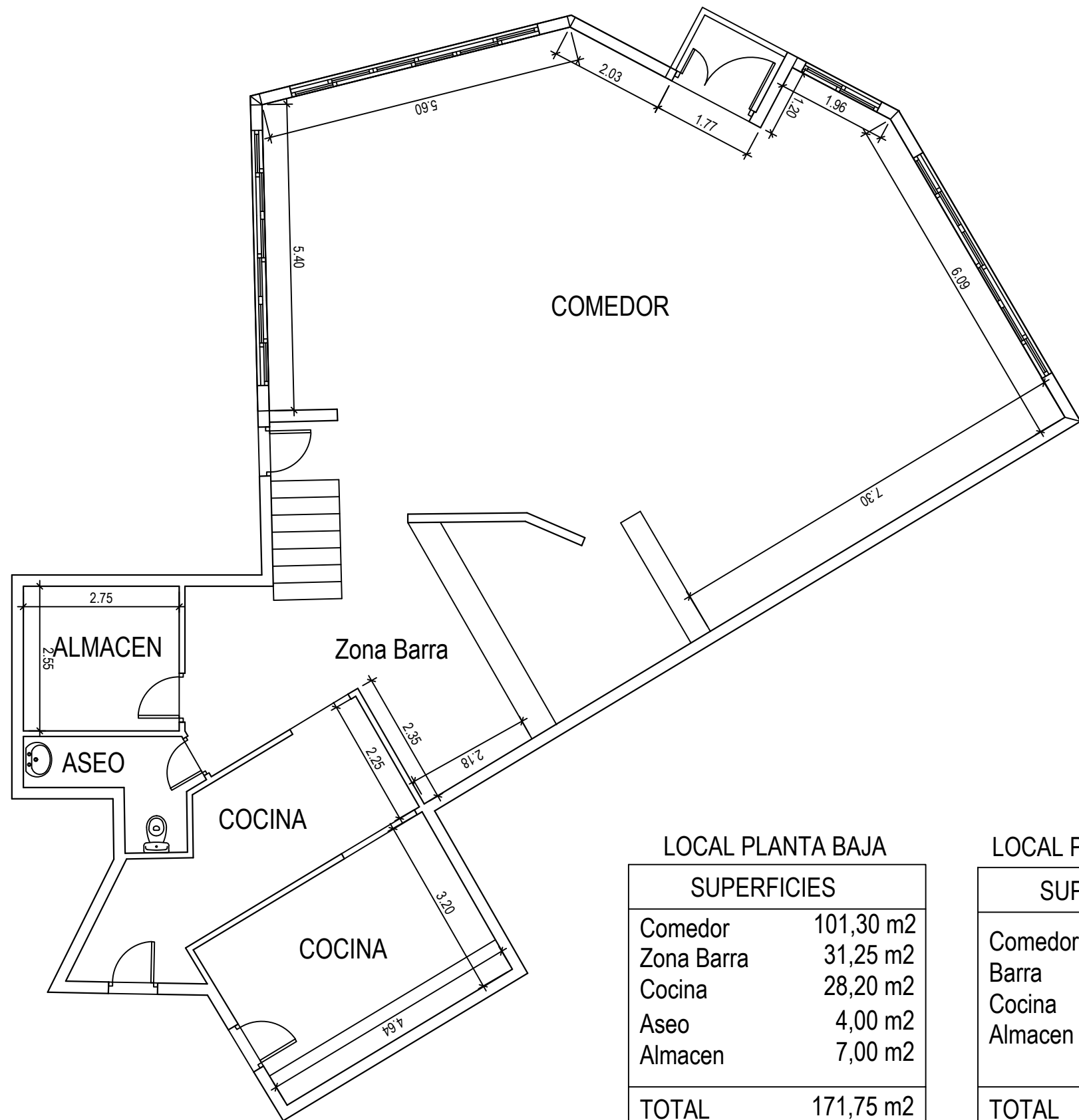
PLANTA BAJA
